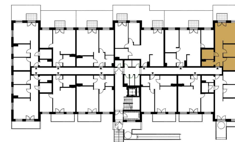
Rzut piętra
