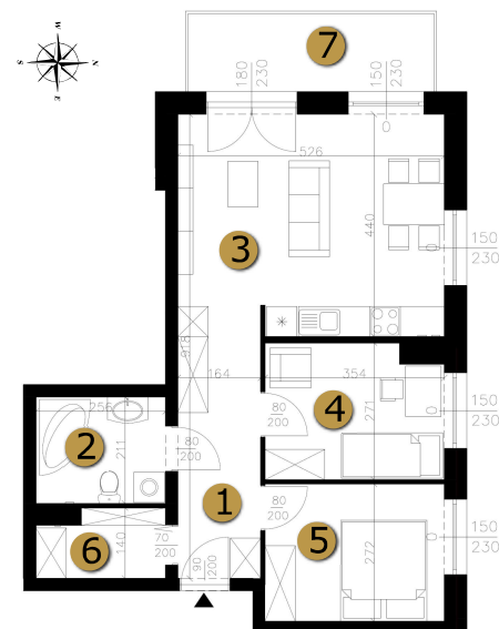
Rzut piętra
